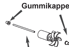
Keramikstab
