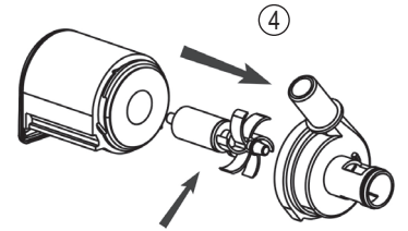
Flügelrad
